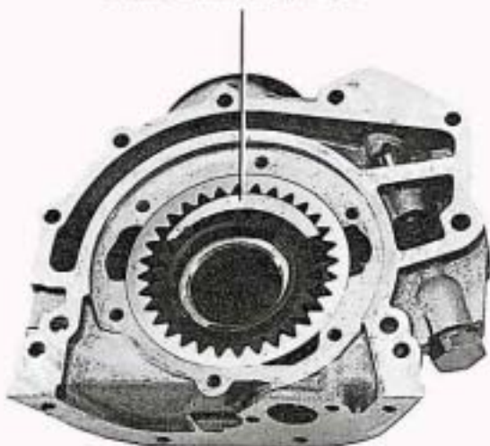
Sichelzahnradpumpe
